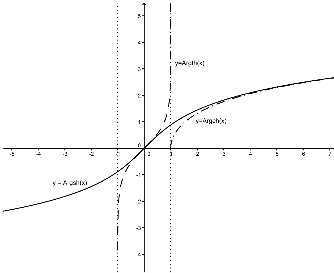
FIGURE 0.1 – Réciproque des fonctions hyperboliques
