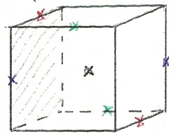
Sous-maille s
