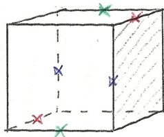
Sous-maille a
